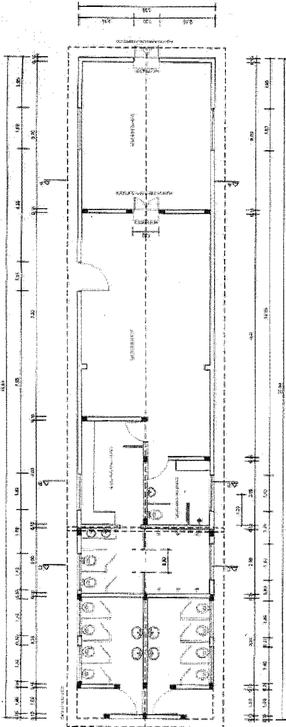
PLANTA DE ALBAÑILERÍA
