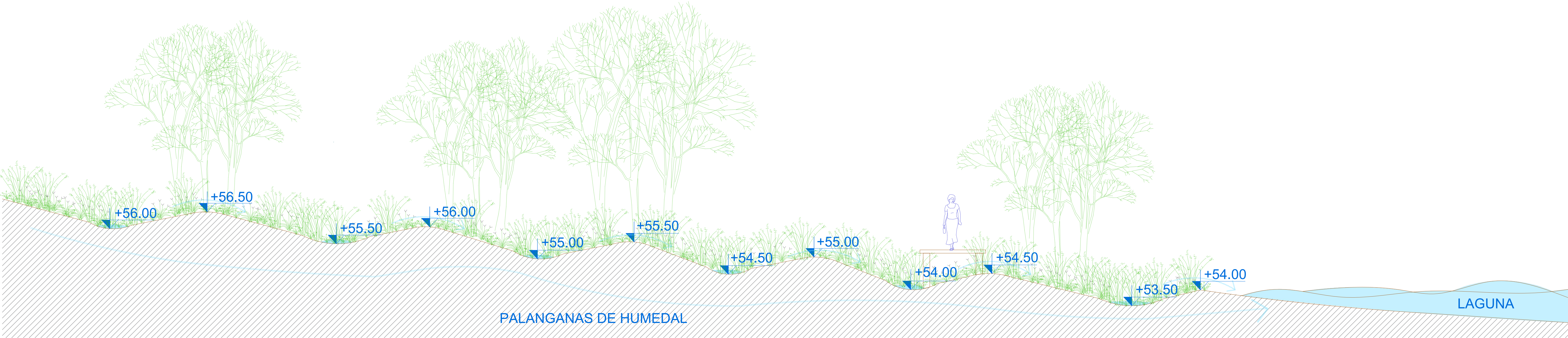
CORTE B-B
