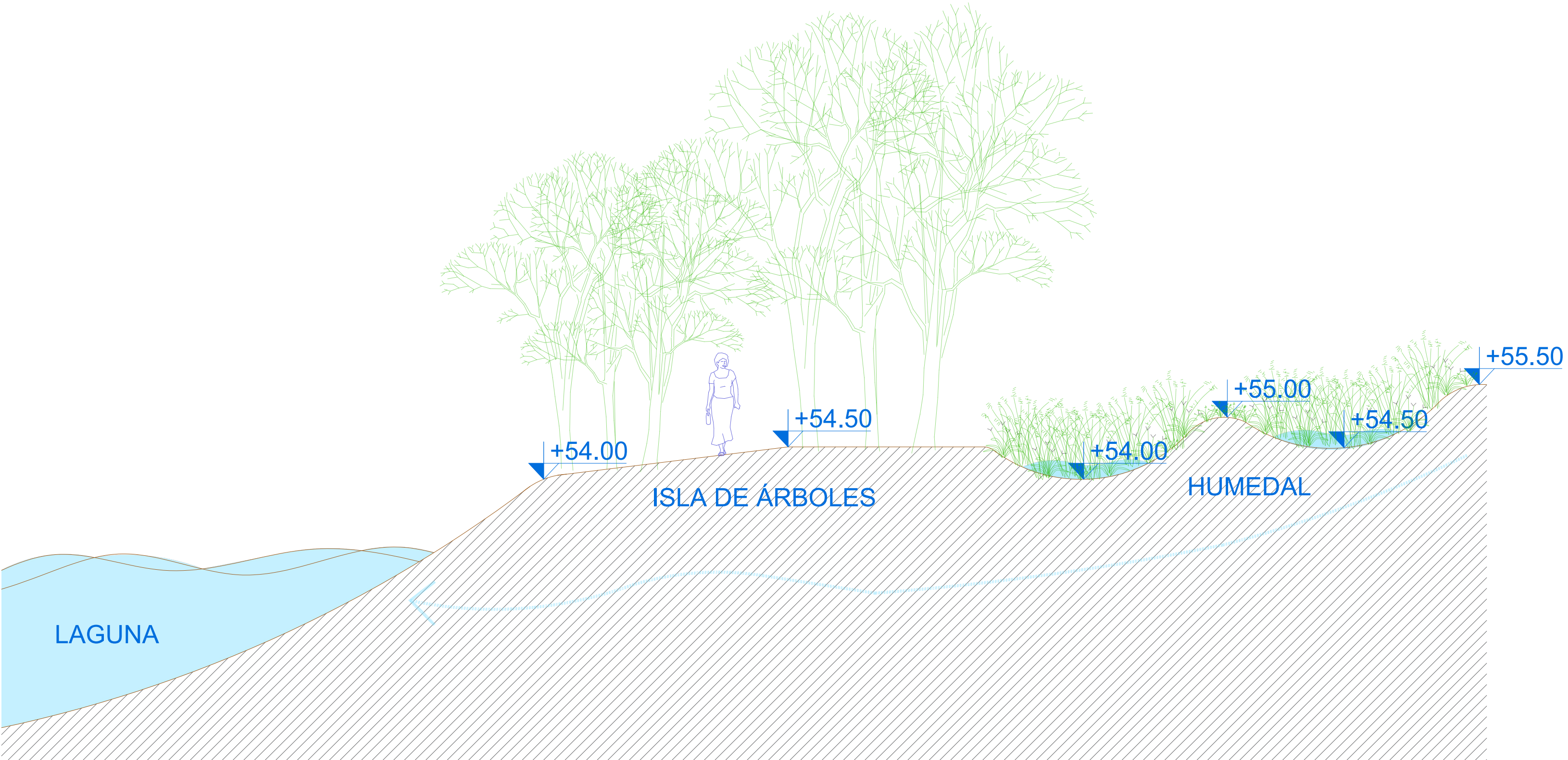
CORTE A-A
